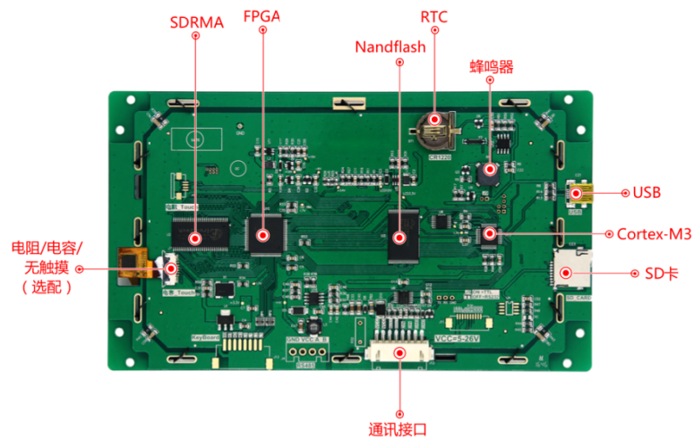
图 1-4 硬件配置图
