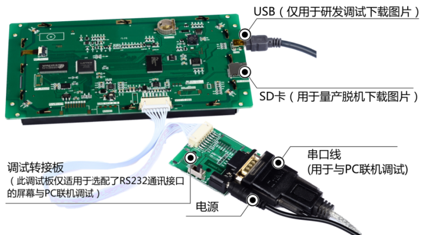
图 1-5 调试工具图
